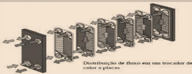
Trocado de calor por placas
