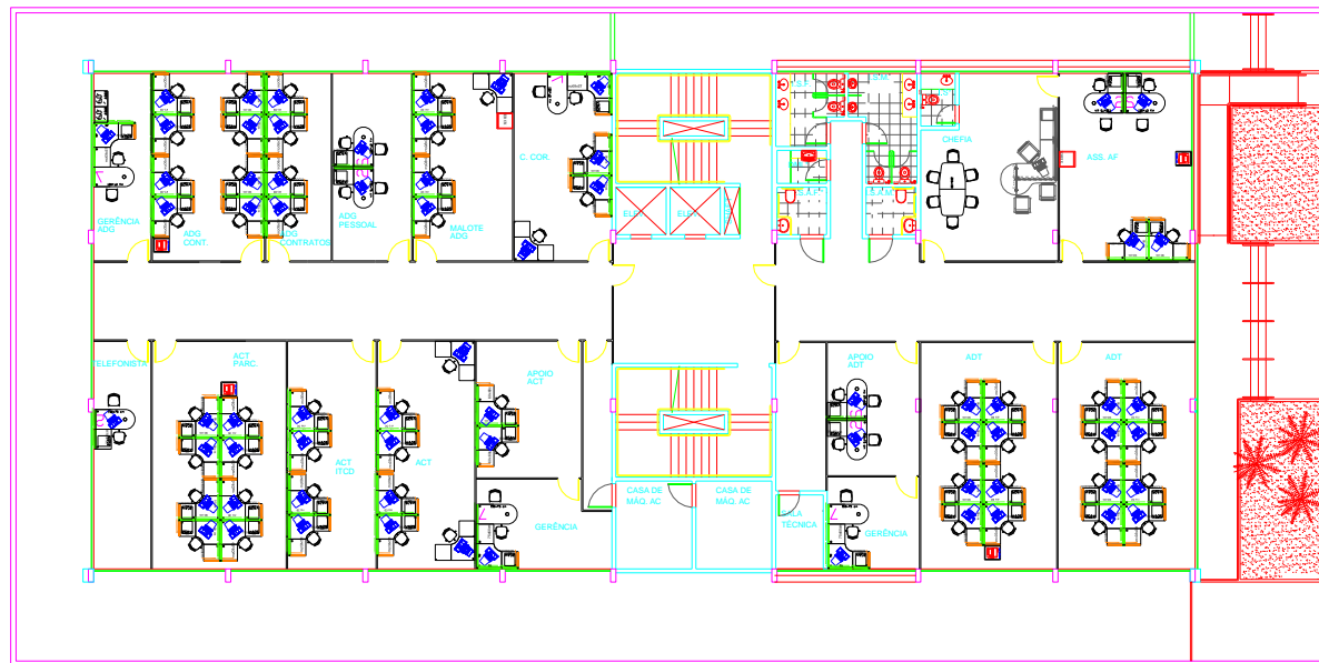
LAYOUT 1º PAVIMENTO
