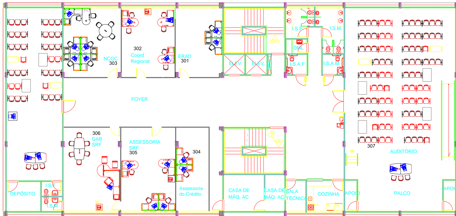
LAYOUT 3 PAVIMENTO
